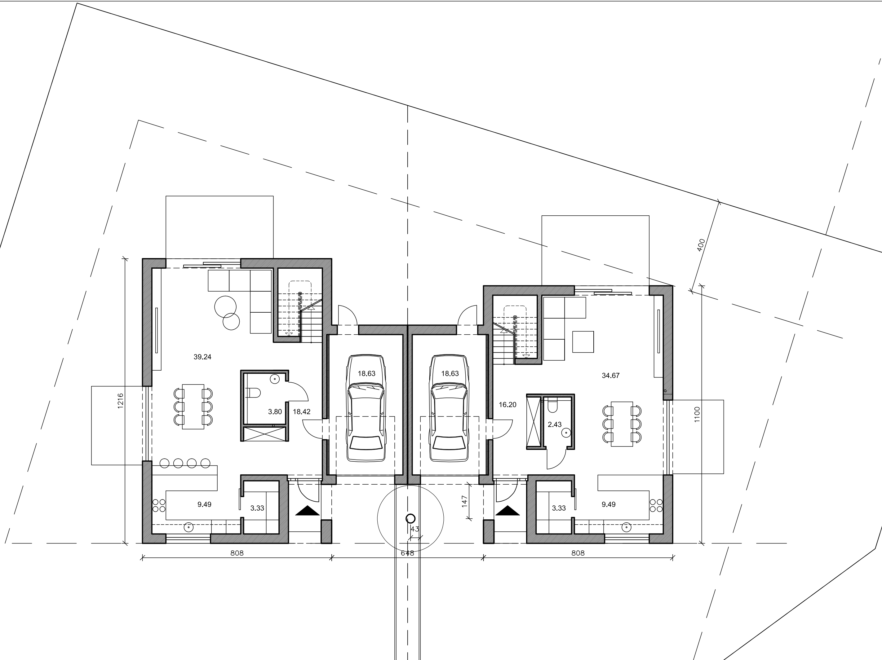
RZUT PARTERU 1:100
